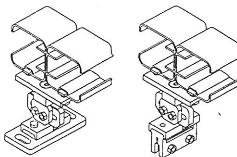
Pose à plat
