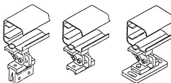
Pose en épine
